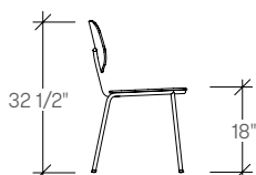
Santé Chair, No Arms (TKAAN)
