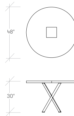
Small Table - ZXRT
