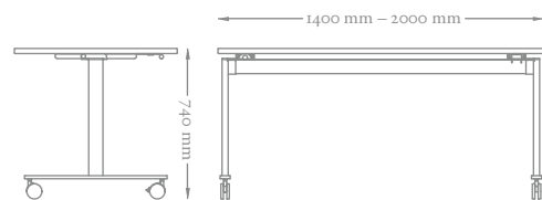
Flip Top Table
