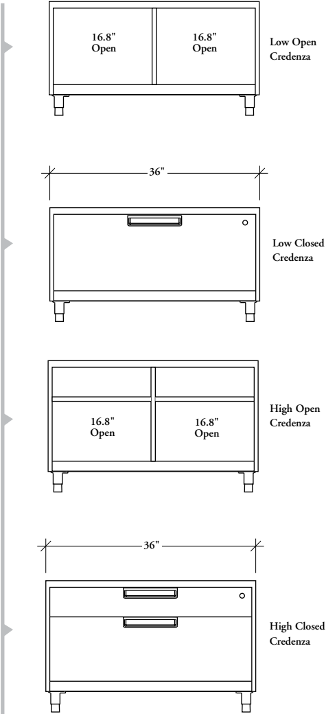
36" Width
